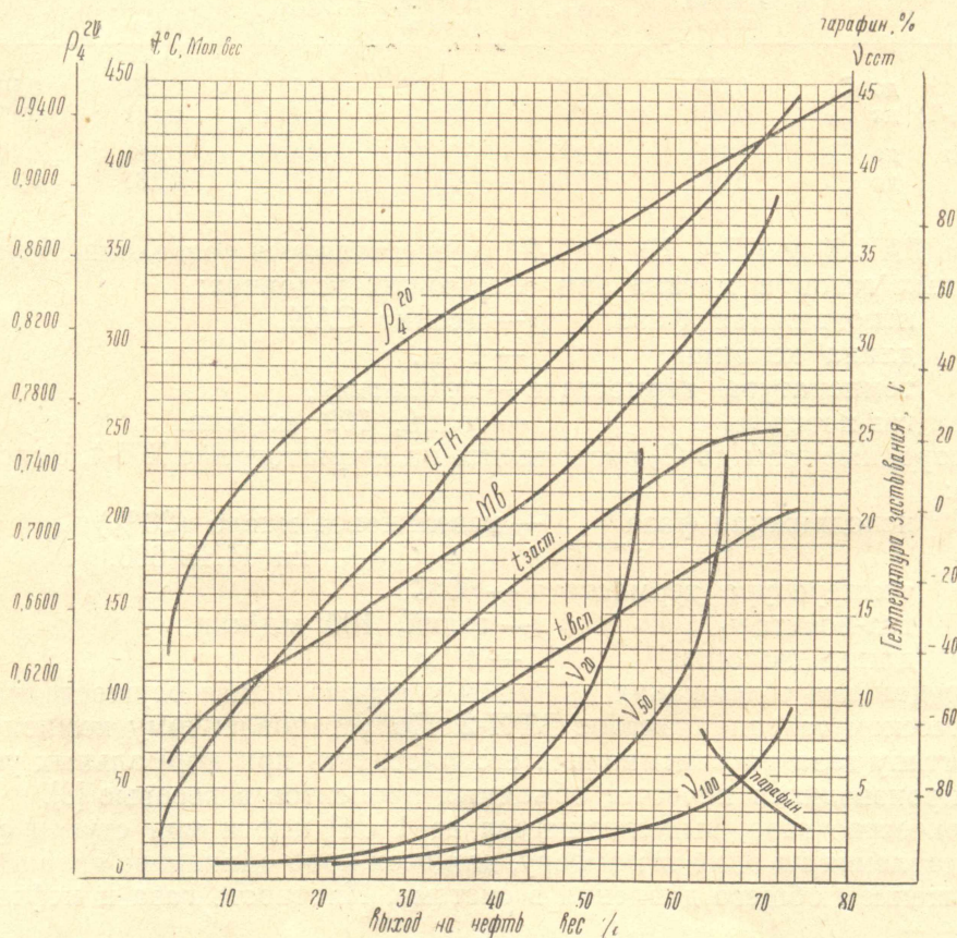
Рис. 1. Кривые разгонки самотлорской нефти
