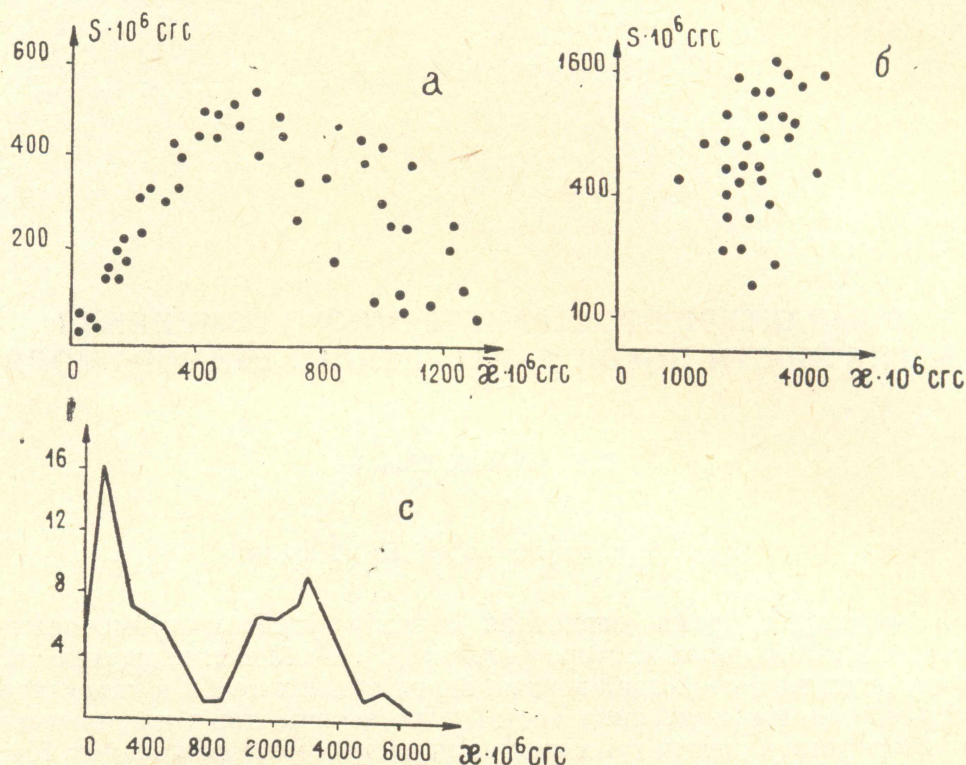
Рис. 1. а) Поле корреляции средней магнитной восприимчивости и ее стандартного отклонения плагногранит-порфиров скв. 602 (рудное поле); б) то же для габбро скв. 551 (периферия месторождения); в) статистический закон распределения магнитной восприимчивости гранодиоритов скв. 579
