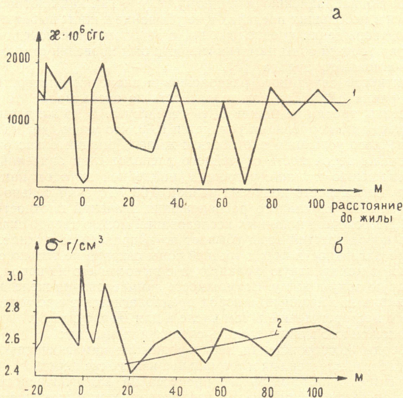
Рис. 3. Графики магнитной восприимчивости (а) и плотности (б) гранодиоритов вкрест простираения одной из жил месторождения; 1 — средняя магнитная восприимчивость гранодиоритов, 2 — линия регрессии плотности пород третьей зоны
