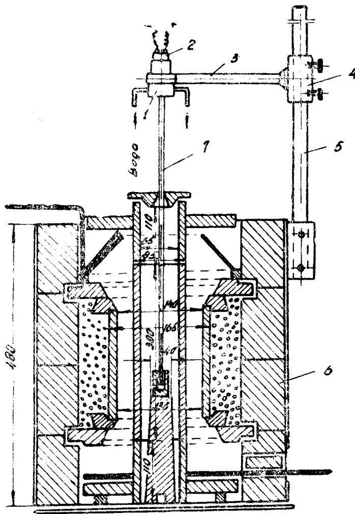
Рис. 1. Конструктивная схема вискозиметра. 1 — водоохлаждаемый экран; 2 — мотор постоянного тока; 3 — кронштейн; 4 — цилиндрическая муфта; 5 — штанги; 6 — криптоловая печь; 7 — шток вискозиметра.
