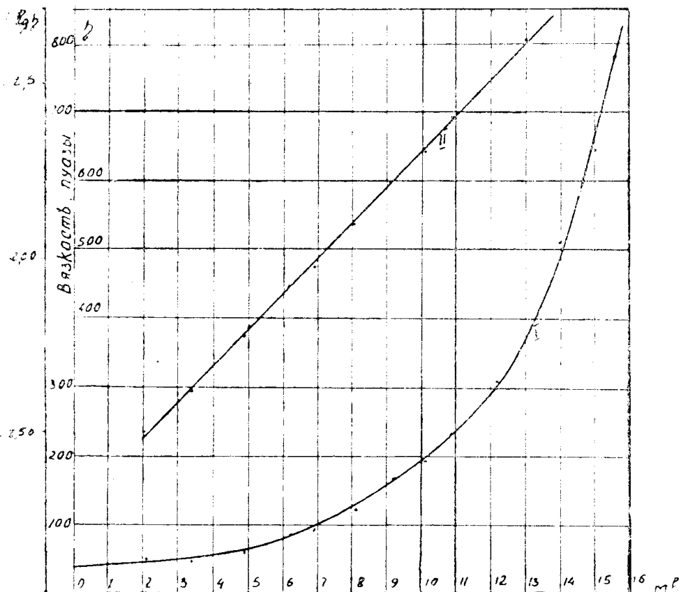
Рис. 3. Тарировочные кривые вискозиметра. I — в обычных координатах; II — в полулогарифмических координатах.
