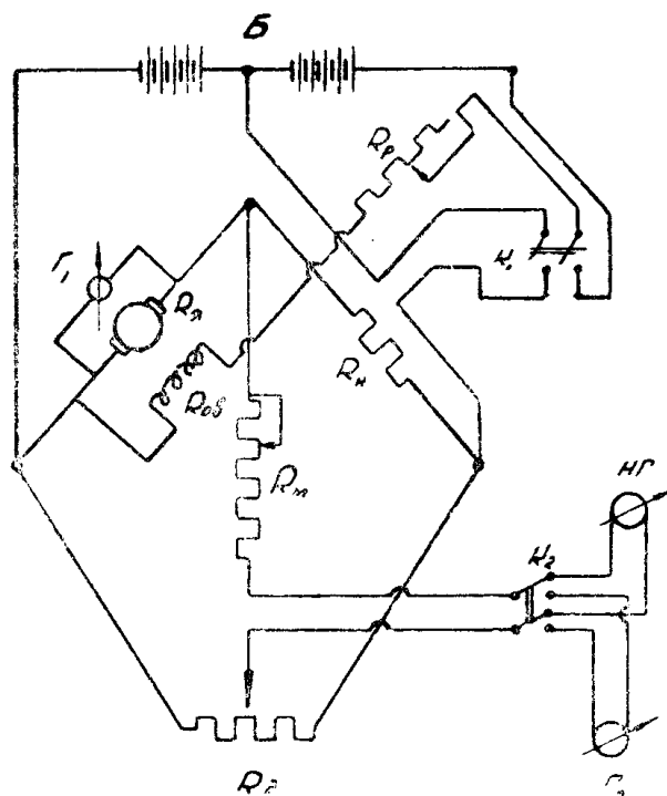
Рис. 2. Электрическая и измерительная схема установки. R_A — якорь мотора; R_{OB} — обмотка возбуждения мотора; R_M — сопротивление для измерения чувствительности прибора; R_K и R_D — постоянное сопротивление моста; R_P — регулировочный реостат; \Gamma_1, \Gamma_2 — гальванометры; НГ — нуль-гальванометр; K_1 — рубильник; K_2 — переключатель.
