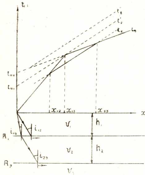
Рис. 1. Возможное соотношение годографов прямых и преломленных волн в случае трехслойной среды. t_1 — годограф прямой волны, t_2 , t_2^1 , t_2^2 — годограф преломленных волн, полученные от границы R_1 при различных отношениях h_2/h_1 , t_3 — годограф преломленных волн, возникших на границе R_2 .
