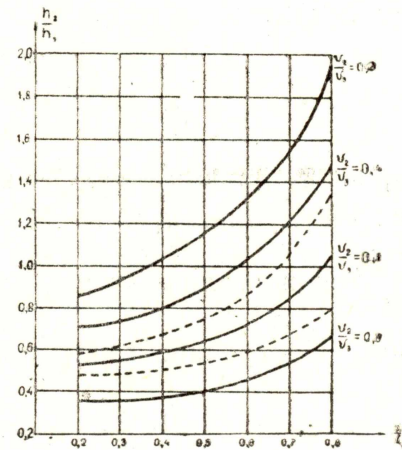
Рис. 2. График для определения минимального значения h_2/h_1 , при котором начинается происходить выпадение пласта в случае горизонтальной трехслойной среды \varphi = \psi = 0 . Пунктиром даны кривые для частного случая: \varphi = 5^\circ , \psi = 0 , v_3/v_1 = 0.6 . Верхняя кривая — по падению границ, нижняя — по восстанию.
