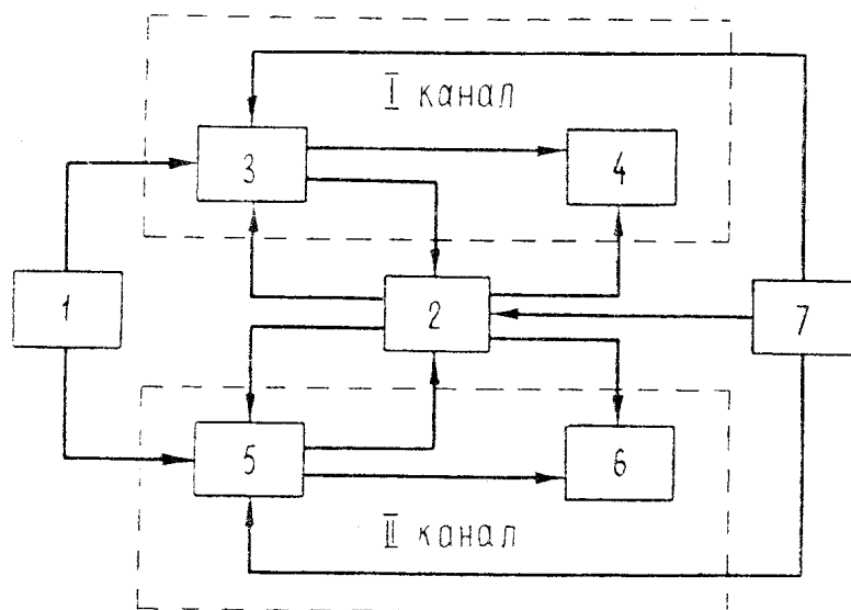
Рис. 2. Блок-схема устройства: 1 — датчик импульсов; 2 — схема сравнения двух переменных величин; 3 и 5 — блоки памяти соответственно I-го и II-го каналов; 4 и 6 — блоки регистрации соответственно I-го и II-го каналов; 7 — программный блок
