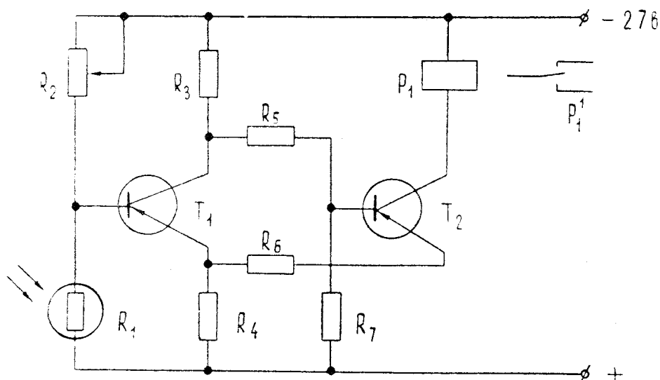
Рис. 1. Принципиальная схема датчика импульсов. T_1 и T_2 — транзисторы типа МП26; R_1 — фотосопротивление типа ФСК-III или ФС-3А; R_2 — R_7 — резисторы соответственно 100; 1,2; 0,27; 1; 0,056; 1,8 ком; P_1 — реле типа РЭС-10, паспорт РС4.524.302
