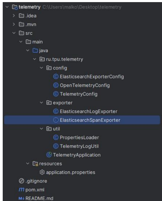
Рис. 2. Структура проекта
