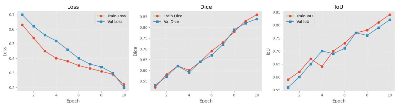
Рис. 6. Метрики и валидация обучения Segnet
