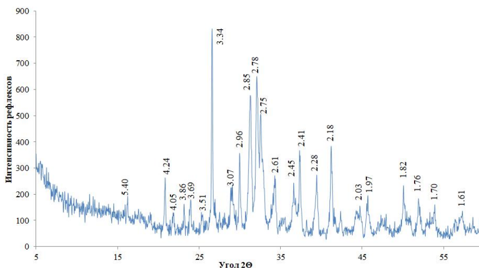
Рис. 7. Рентгеновская дифрактограмма неизмельчённой кремнисто-карбонатной породы, обожжённой при 1100 °С Fig. 7. X-ray diffraction pattern of unground siliceous-carbonate rock fired at 1100 °C
