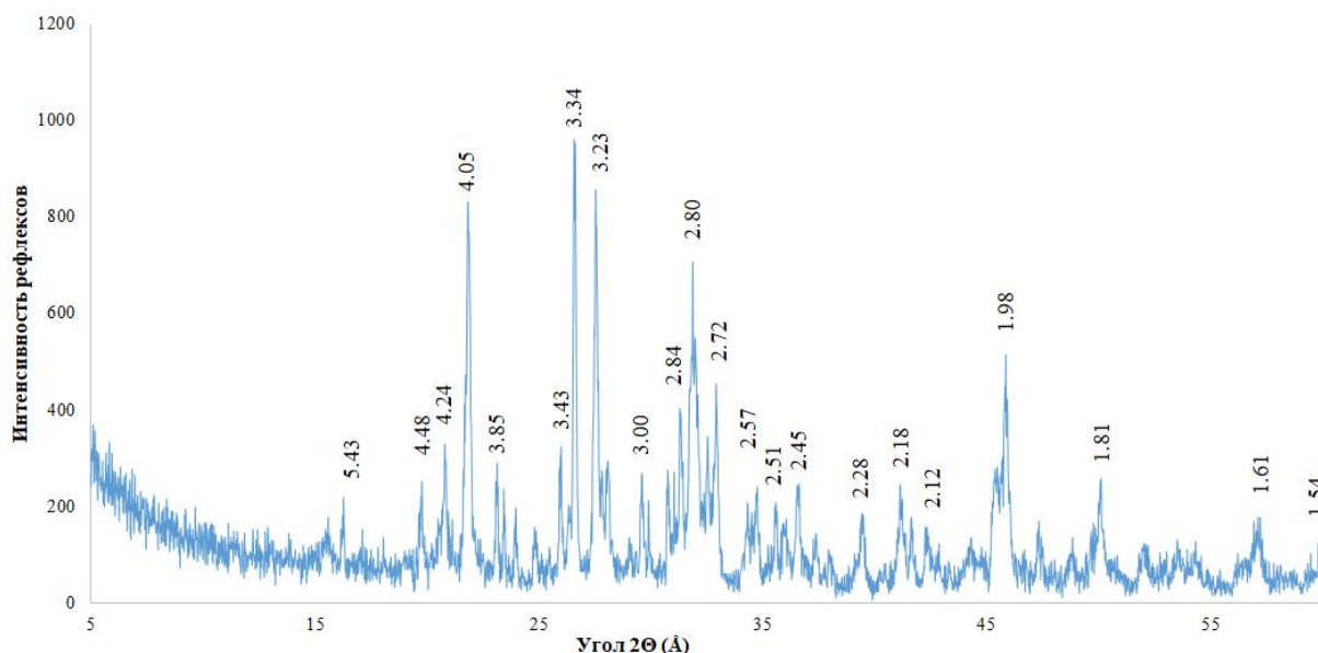
Рис. 3. Рентгеновская дифрактограмма синтетического волластонита на основе кварцевого песка и известняка Fig. 3. X-ray diffraction pattern of synthetic wollastonite based on quartz sand and limestone
