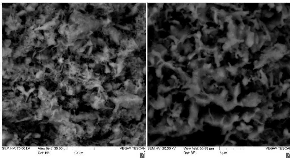
Рис. 10. Снимки синтезированного волластонита, выполненные под электронным микроскопом Fig. 10. Pictures of synthesized wollastonite made under an electron microscope
