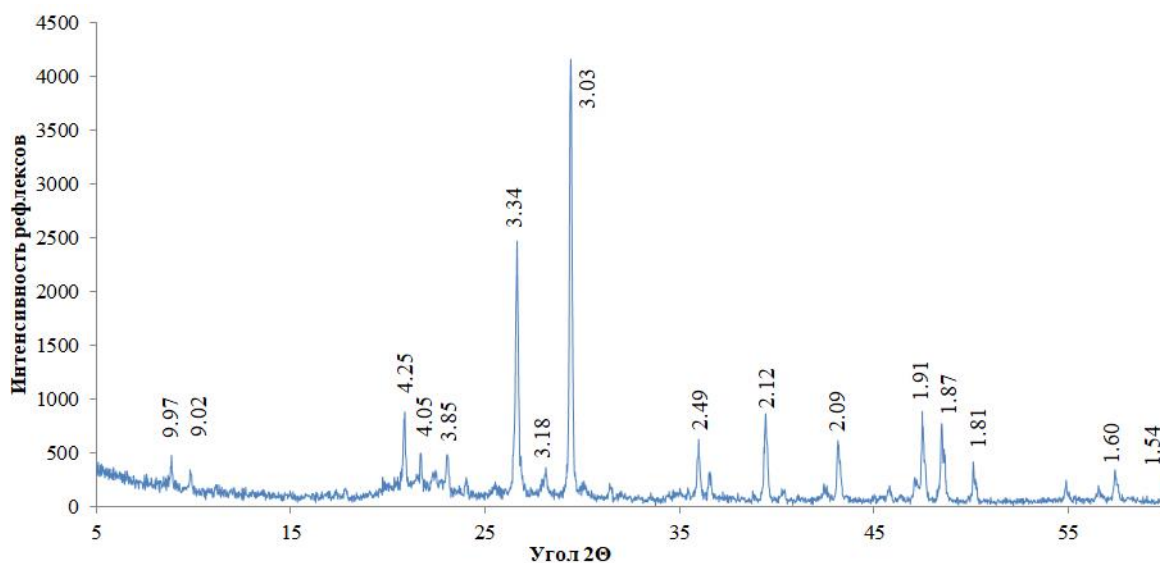
Рис. 5. Рентгеновская дифрактограмма кремнисто-карбонатной породы
