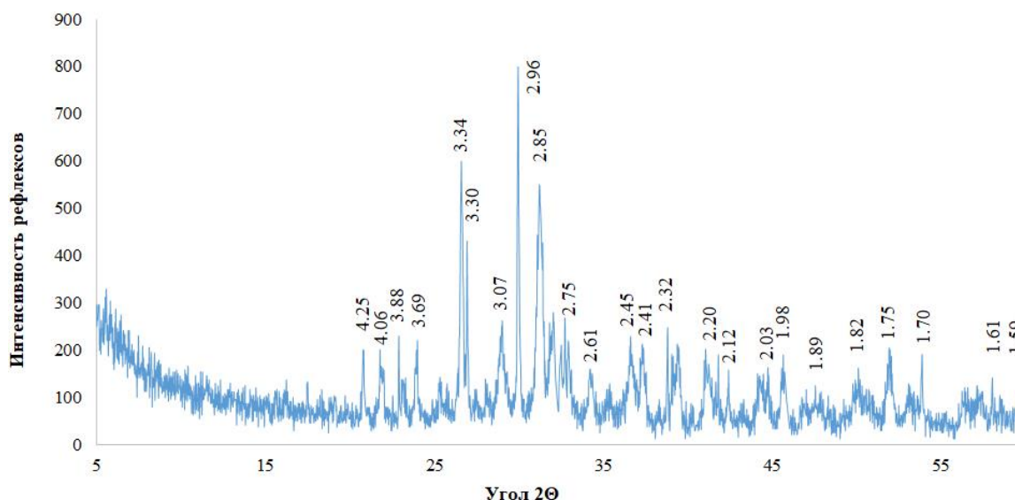
Рис. 9. Рентгеновская дифрактограмма измельчённой кремнисто-карбонатной породы, обожжённой при 1100 °С
