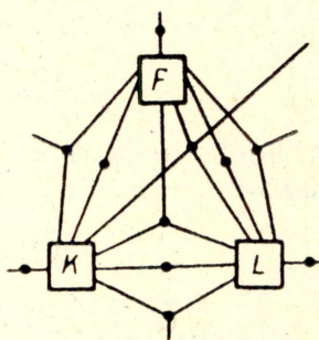
Рис. 3. К теореме 1
