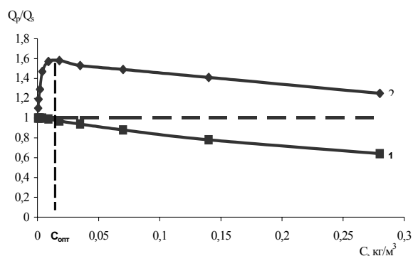
Рис. 1. Зависимость относительных скоростей от концентрации растворов полигексена в гептане: 1) ламинарное и 2) турбулентное течение
