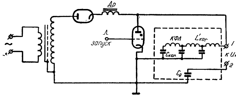
Рис. 1. Принципиальная схема импульсного модулятора с комбинированным накопителем
