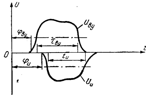
Рис. 4. Волновая диаграмма импульсов: U_{by} — импульс инфлектора, U_{и} — импульс электронной пушки, \varphi_{by} и \varphi_{и} — задержки (фазы) соответствующих импульсов
