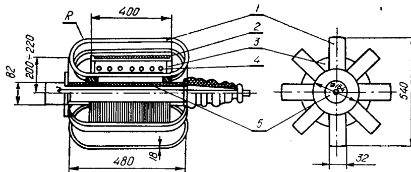
Рис. 2. Эскиз конструктивного объединения электронной пушки торцового типа и импульсного трансформатора
