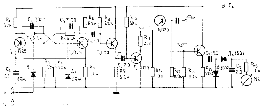
Рис. 1. Принципиальная схема измерителя энергии
