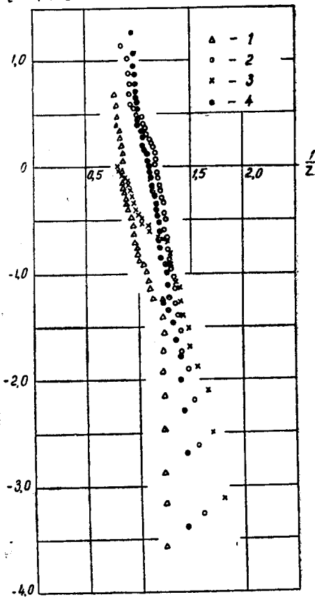
Рис. 1. Зависимость \ln[-\ln P(\tau)] - \ln Z от \frac{1}{Z} для кабелей марки СБ при различных E_{\text{max}}
