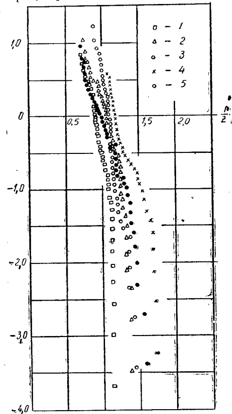
Рис. 2. Зависимость \ln[-\ln P(\tau)] - \ln Z от \frac{1}{Z} для образцов фазы кабеля марки АСБ при различных E_{\text{max}}
