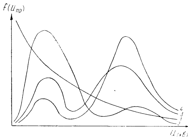
Рис. 1. Кривые распределения U_{пр} проводов, поврежденных при укладке обмотки в пазы статора. Электроды: 1 — графит, 2 — ртуть, 3 — дробь, 4 — плоский металлический электрод
