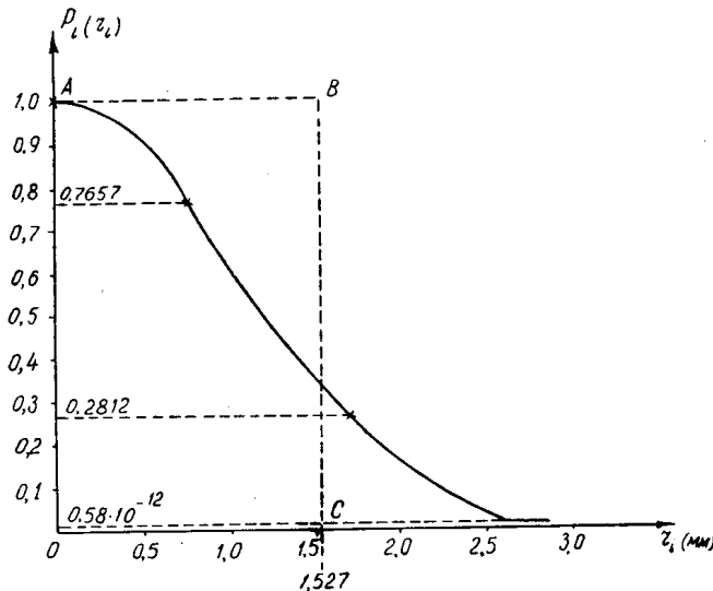
Рис. 4. Зависимость вероятности выявления дефектов от расстояния дефекта до плоского электрода
