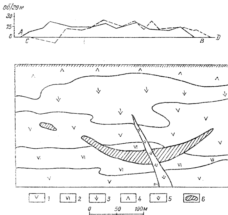
Рис. 2. График биофизической аномалии над медноколчеданным месторождением Летнее: 1 — подушечная лава диабазов; 2 — подушечная лава спилитов; 3 — глыбовая лава диабазов; 4 — подушечная лава порфиров; 5 — жильный диабаз; 6 — сульфиды. АВ — график биофизической аномалии, выявленной при работе с латунной рамкой. СД — график биофизической аномалии — со стальной рамкой.
