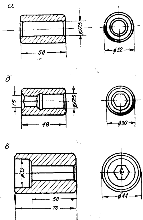
Рис. 2. Конструкции концевых букс рубильно-клепальных молотков: а) цилиндрическая; б) комбинированная; в) граненая.
