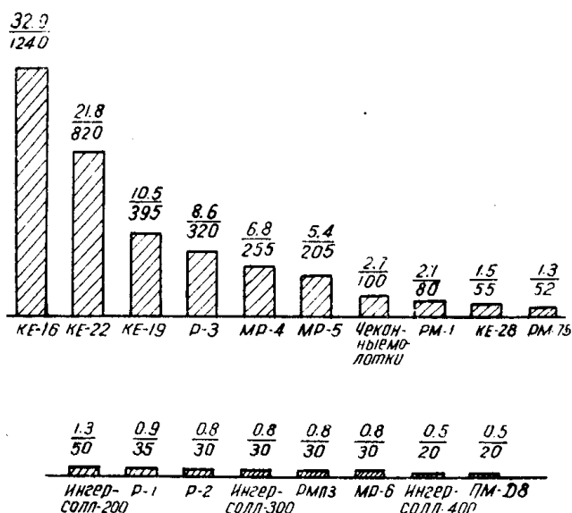
Рис. 1. Распространение различных типов молотков, эксплуатируемых на обрубке и зачистке литья (3767 молотков) в процентах/шт.
