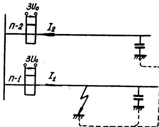
Рис. 1. Распределение тока нулевой последовательности при замыкании на землю в сети с изолированной нейтралью.
