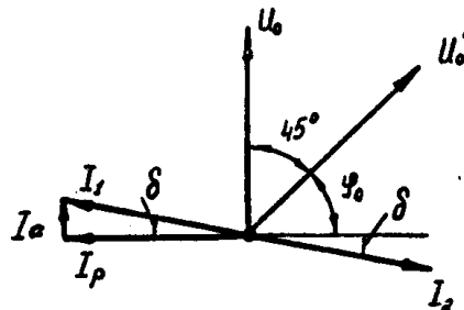
Рис. 4. Векторная диаграмма токов и напряжений при замыкании на землю в сети рис. 1.
