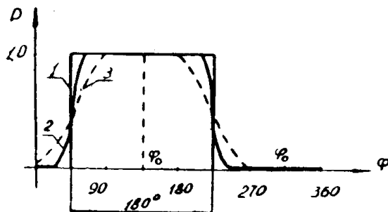
Рис. 3. Характеристики управляемости фазой колебаний параметрона. P — вероятность возникновения параметрических колебаний с фазой +90^\circ ; \varphi — угол сдвига фаз между напряжением подмагничивания и током замыкания; 1 — теоретическая кривая; 2, 3 — экспериментальные кривые соответственно при I_{02} > I_{03} .
