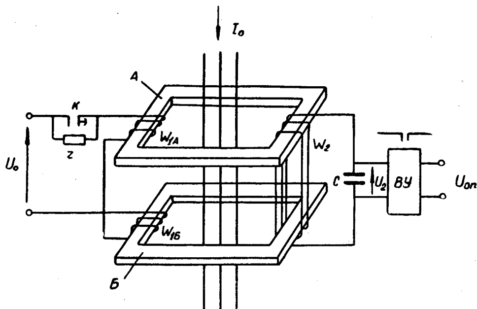
Рис. 2. Принцип устройства параметрона. А и Б — два одинаковых замкнутых магнитопровода; w_{1A} и w_{1B} — обмотки подмагничивания с одинаковым количеством витков; w_2 — вторичная обмотка; C — конденсатор; K — управляемый контакт; z — сопротивление; U_0 — напряжение подмагничивания; I_0 — ток замыкания на землю; ВУ — выходное устройство, представляющее собой орган фазовой селекции; U_{он} — опорное напряжение.
