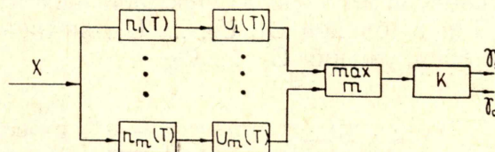
Рис. 1. \chi — канал обработки радиометрической информации; n_j(T) , ( j=1, 2, \dots, m ) — сумматор числа электрических импульсов за время T ; U_j(T) , ( j=1, 2, \dots, m ) — блок вычисления статистики U ; \left(\frac{\max}{m}\right) — блок поиска максимума; K — порог обнаружения; \gamma_1 — решение о наличии сигнала от дефекта; \gamma_0 — решение об отсутствии сигнала от дефекта.
