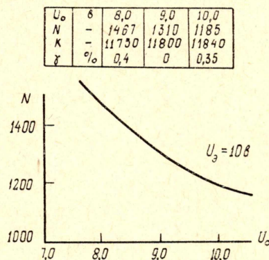
Рис. 7. Характеристика управления коэффициентом преобразования.
