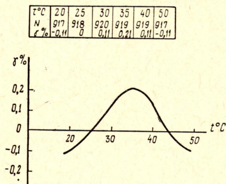
Рис. 6. Испытания ГСН на температурную нестабильность.
