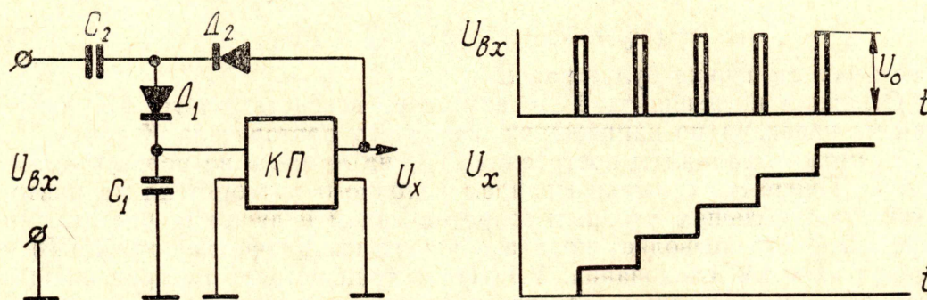
Рис. 2. Генератор ступенчатого напряжения на основе емкостного делителя с катодным повторителем.
