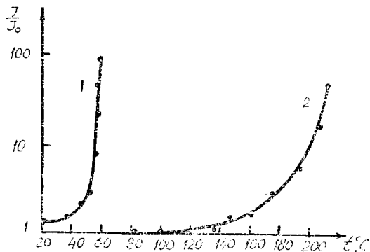
Рис. 1. Зависимость тока от температуры: 1) Ag — стекло — Al, 2) Ag — кристалл NaCl.
