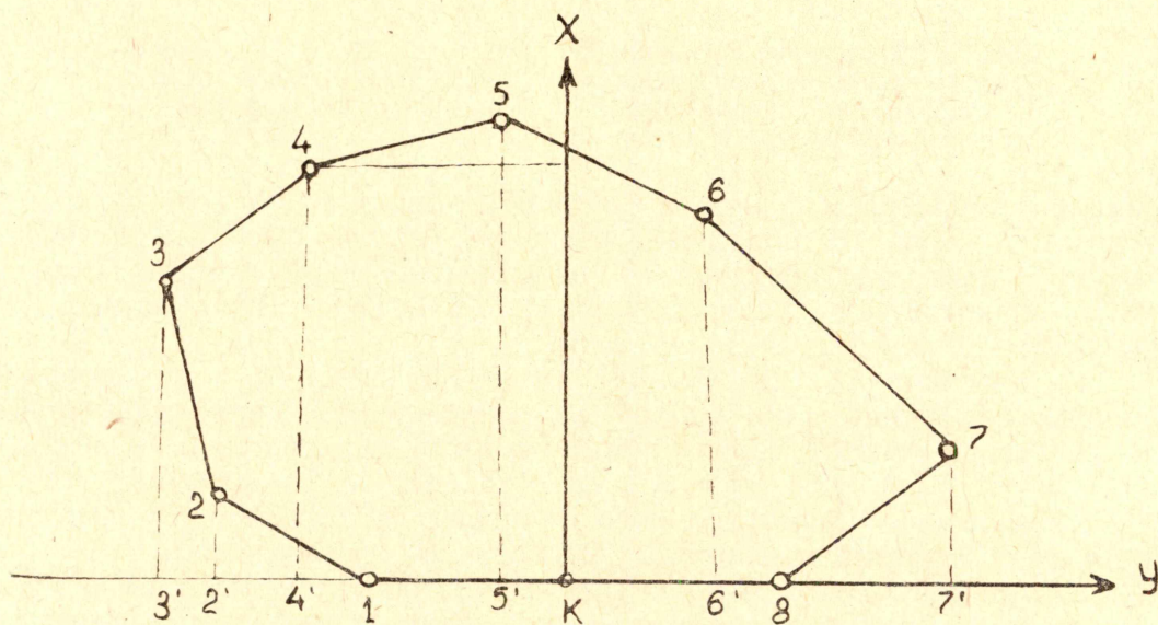
Рис. 10. Схема теодолитного хода при сбойке горной выработки.
