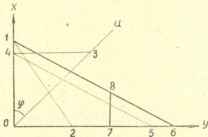
Рис. 2. Определение для угла значения X графическим путем.
