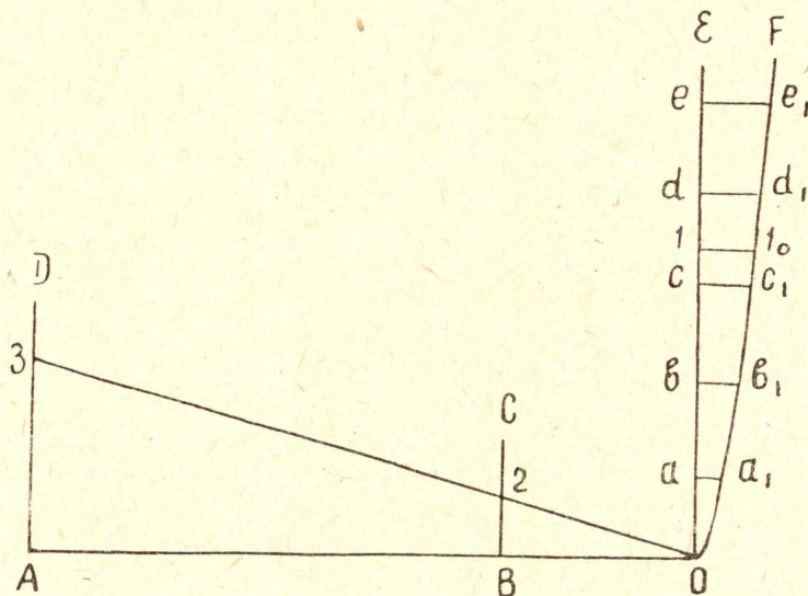
Рис. 6. Определение ошибки m_l графическим способом.
