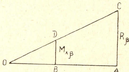
Рис. 11. Определение ошибки смыкания забоев горной выработки в зависимости от ошибки измерения углов графическим путем.
