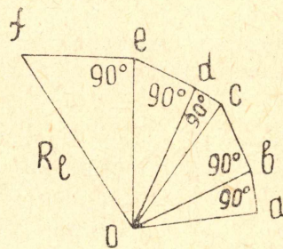
Рис. 8. Прямоугольный полигон для определения R_l .
