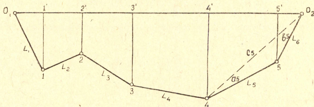
Рис. 1. Схема теодолитного хода при ориентировке через два вертикальных ствола.
