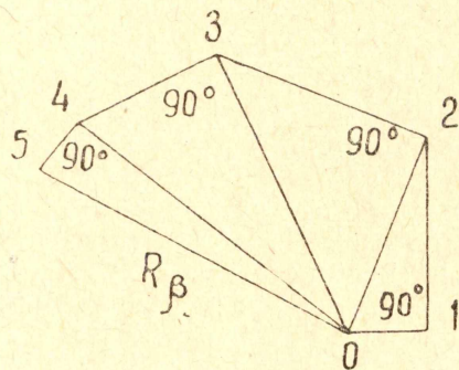
Рис. 4. Прямоугольный полигон для определения R_{\beta}
