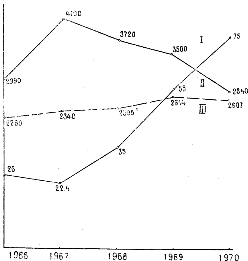
Рис. 1. Производительность буровых установок, процент поискового бурения и средние глубины скважин по Томскому территориальному геологическому управлению за 1966—1970 гг.
