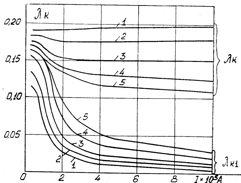
Рис. 3. Зависимость коэффициента проводимости по коронкам зубцов \lambda_k и коэффициента проводимости \lambda_{k1} от тока в пазах I
