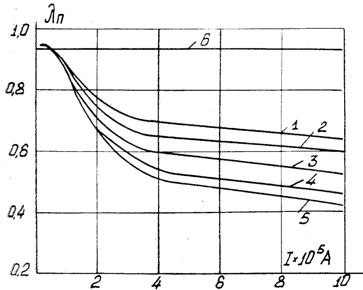
Рис. 2. Зависимость коэффициента проводимости пазового рассеяния \lambda_{\pi} от тока в пазу I
