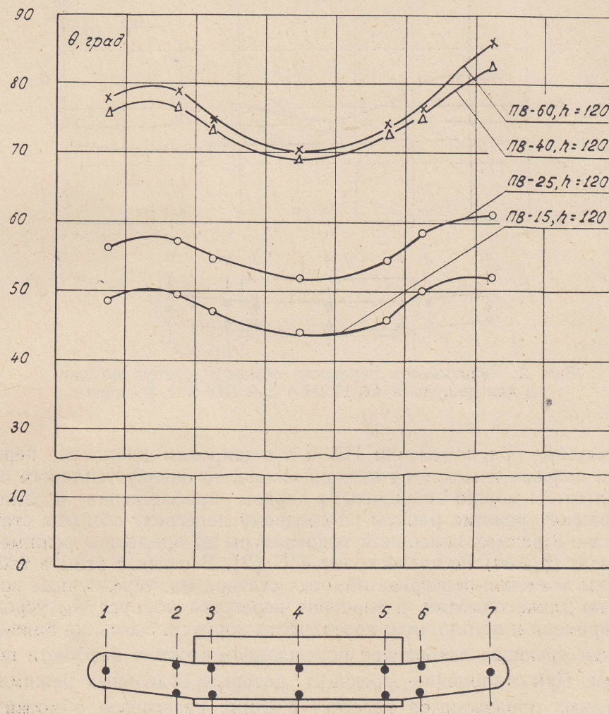
Рис. 1. Зависимость перегрева обмотки статора по длине для двигателя 4А-112М-4 при h=\text{var} , PB=\text{const}
