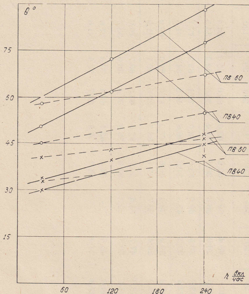
Рис. 3. Влияние числа включений на перегрев обмотки статора \bullet и корпуса \times при различных ПВ: — — — для двигателя 4A-112M-4; — — — для двигателя 4A-112M-6
