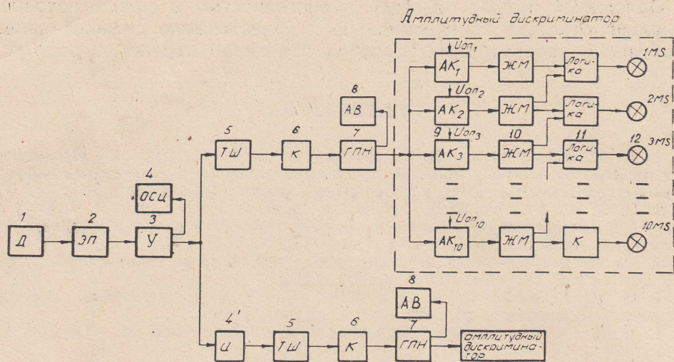
Рис. 1. Полная функциональная схема прибора
