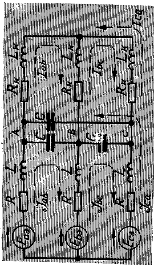
Рис. 3. Схема замещения инвертора.
