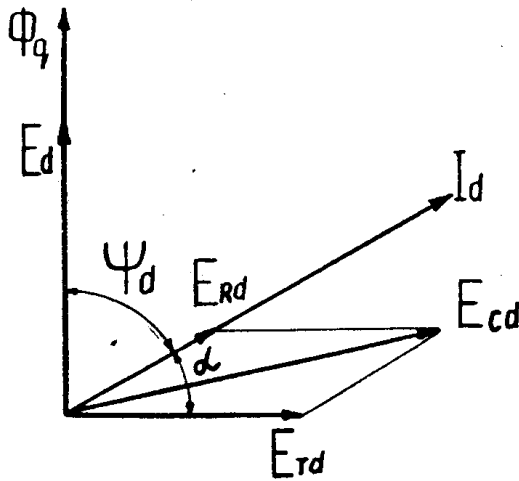
Рис. 3. Векторная диаграмма э. д. с. коммутируемых секций продольной цепи.
