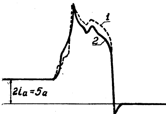
Рис. 6. Кривые тока коммутируемых секций продольной цепи, питаемой постоянным и переменным током, при отключенных дополнительных полюсах: 1 — переменный ток частоты 50 Гц, 2 — постоянный ток.
