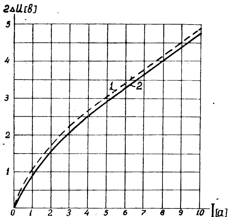
Рис. 4. Статические вольт-амперные характеристики щеток ЭГ-8: 1 — переменный ток частоты 50 Гц, 2 — постоянный ток.
