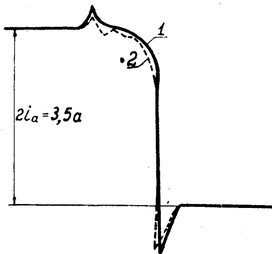
Рис. 5. Кривые тока коммутируемых секций поперечной цепи, питаемой постоянным и переменным током: 1 — переменный ток частоты 50 Гц, 2 — постоянный ток.
