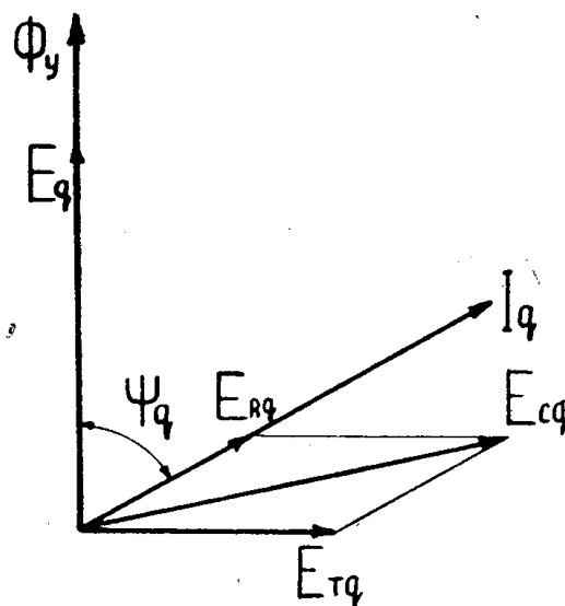
Рис. 2. Векторная диаграмма э. д. с. коммутируемых секций поперечной цепи.
