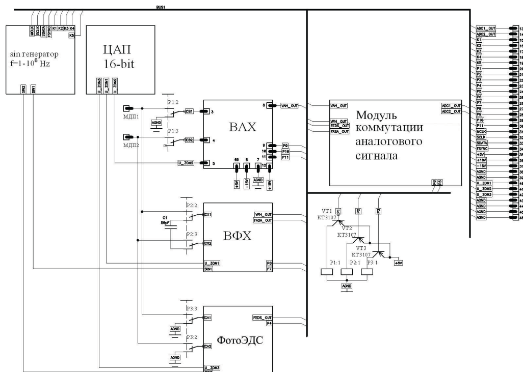
Рис. 2. Структурная схема блока преобразования параметров
