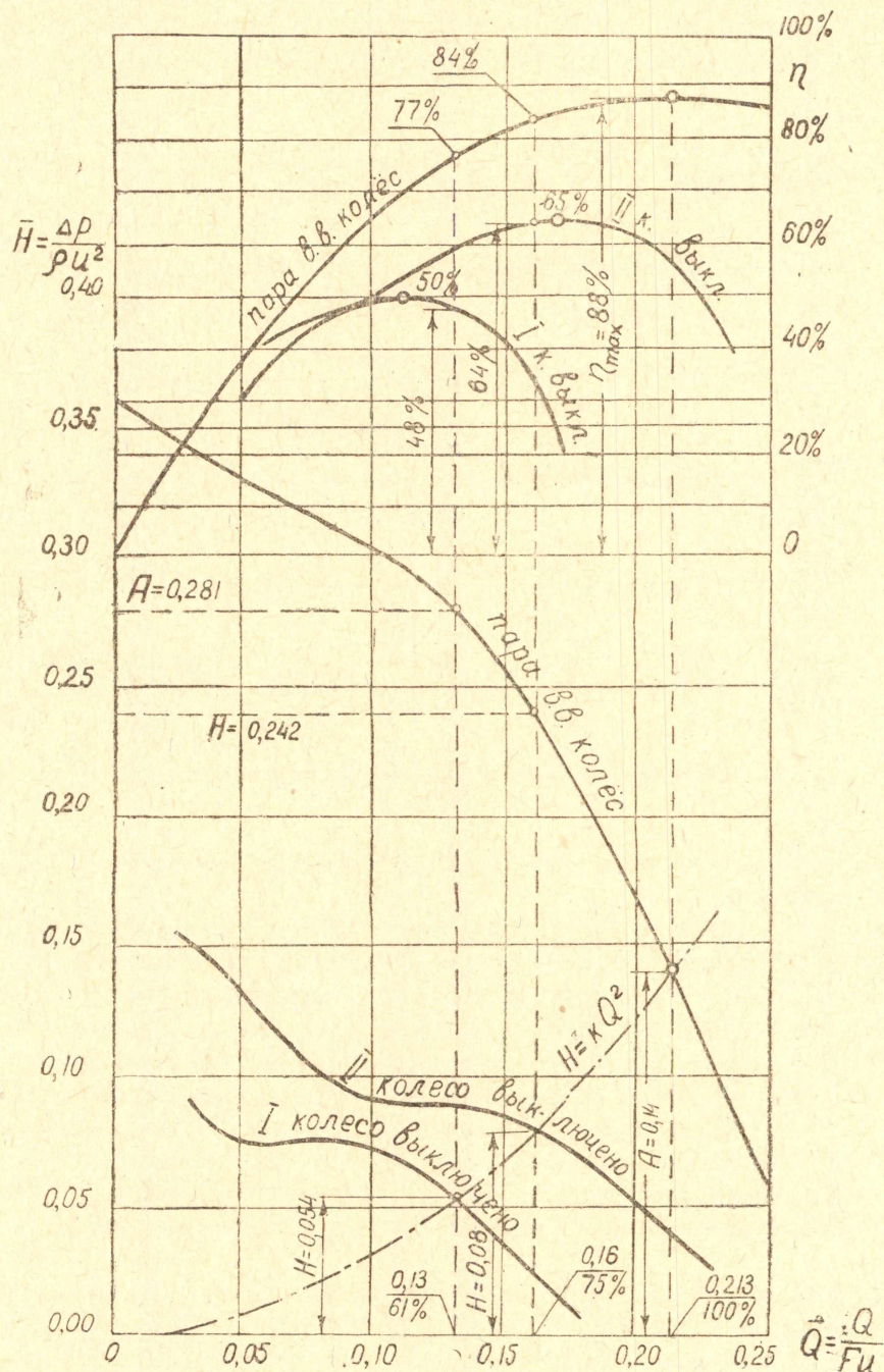
Рис. 8. Выключение приводов первого и второго встречно вращающихся осевых колёс.
