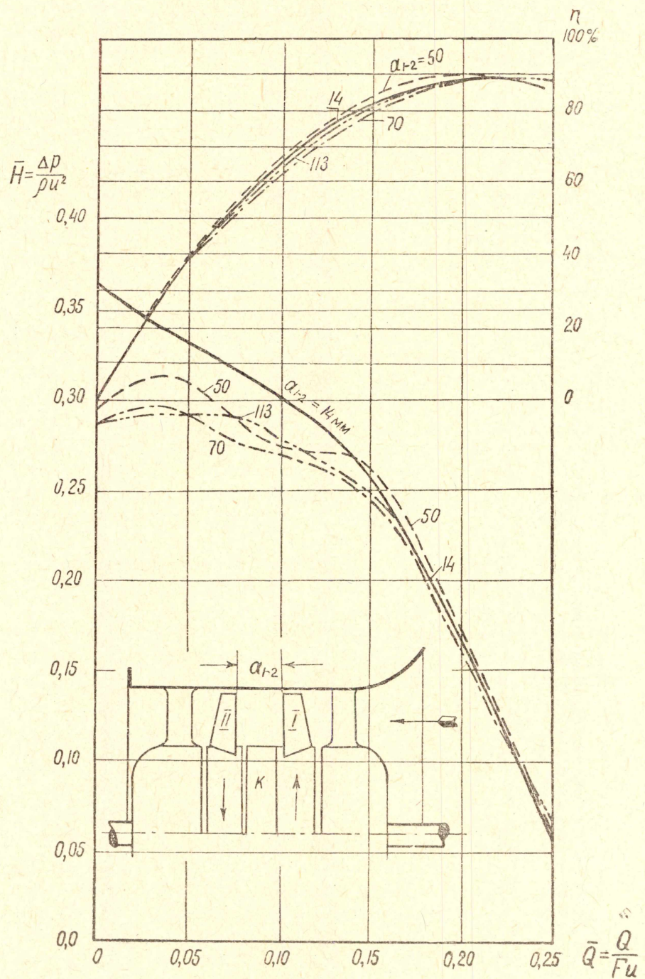
Рис. 6. Влияние осевого расстояния между парой встречновращающихся осевых колес на их характеристики.
