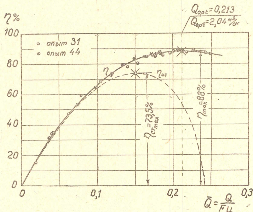
Рис. 3. К. п. д. экспериментальной модели ВДВ-Э.
