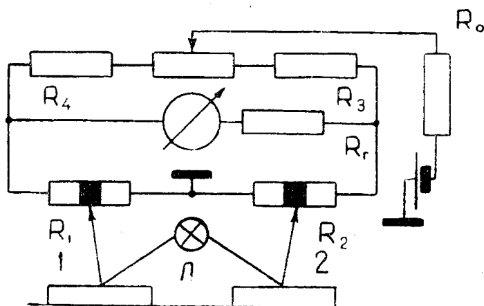
Рис. 2. Схема измерительного моста. R_1 , R_2 — фотосопротивления ФС-К1; R_3 , R_4 — плечи моста; R_r — сопротивление рамки микроамперметра, равное 100 ом; R_0 — внутреннее сопротивление источника питания; 1 — исследуемая проба; 2 — эталонная проба; Л — осветительная лампа.
