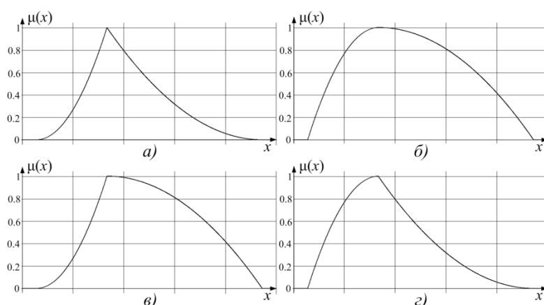
Рис. 1. Формы функций принадлежности с учетом дополнительных условий (4)–(7)
