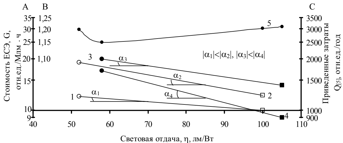
Рис. 2. Сравнение в качестве критерия стоимостей: 1) приведенной, отн.ед./год, ламп ДРЛ 250 vs ДНаТ 150; 2) ЕСЭ, отн.ед./Млм·ч, тех же ламп; 3) приведенной, отн.ед./год, ламп ДРЛ 400 vs ДНаТ 250; 4) ЕСЭ, отн.ед./Млм·ч, тех же ламп. 5) коэффициент Q_{[5]}/G\Phi T
