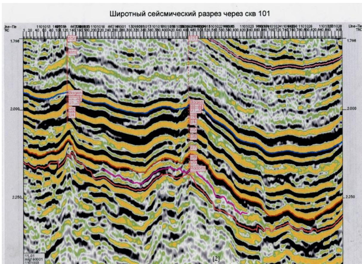
Рис. 3. Сейсмический разрез через скважину 101 Восточно-Хохряковского месторождения Ханты-Мансийского автономного округа
