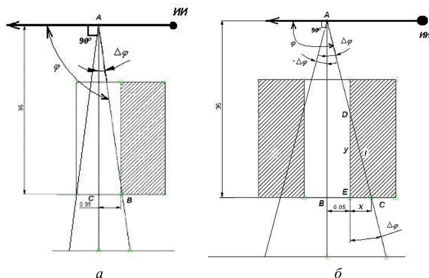
Рис. 5. Геометрия системы прохождения излучения через коллиматор: а – прохождение ИИ в проводнике без потерь; б – прохождение ИИ через материал поглотителя
