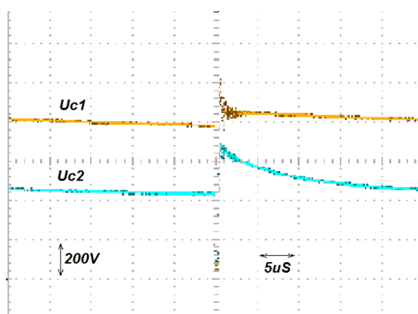
Рис. 8. Осциллограммы напряжений на четырех транзисторах до коррекции: U_{c1} – напряжение на четырех транзисторах; U_{c2} – на двух
