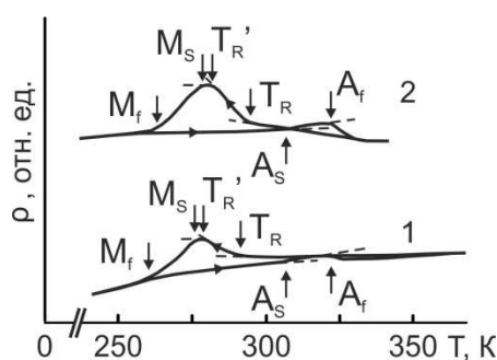
Рис. 1. Зависимость электросопротивления от температуры для [1\bar{2}3] монокристаллов Ti-49Ni-1Fe: 1 – без водорода; 2 – после наводороживания в течение 2 ч. в H_2SO_4 при T=295K и j=1400 A/m^2
