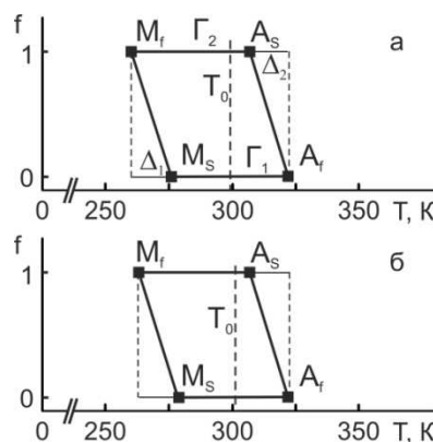
Рис. 2. Термические гистерезисы для [1\bar{2}3] монокристаллов Ti-49Ni-1Fe: 1 – без водорода; 2 – после наводороживания в течение 2 ч. в H_2SO_4 при T=295K и j=1400 A/m^2
