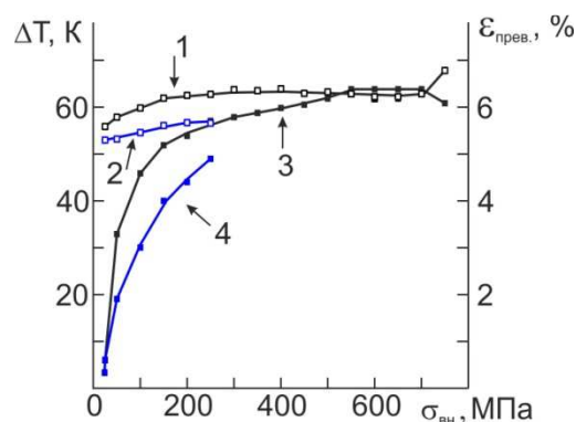
Рис.4. Зависимость термического гистерезиса (1,2) и величины ЭПФ (3,4) от уровня приложенных внешних напряжений для [\bar{1}23] монокристаллов Ti-49Ni-1Fe при деформации растяжением: 1,3 - без водорода, 2,4 - после наводороживания в течение 2 ч. в H_2SO_4 при T=295K и j=1400 A/m^2
