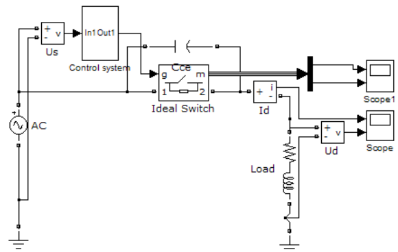
Рис. 2. Схема с Ideal Switch.
