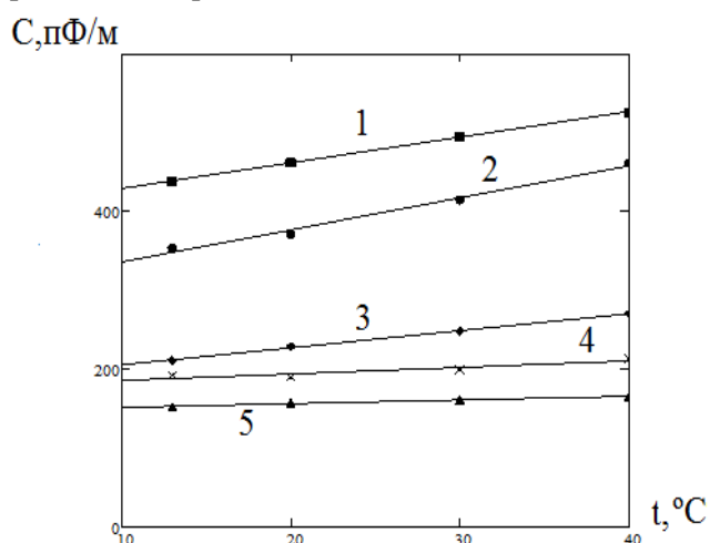
Рис 3. «Зависимость влияния температуры воды на результат измерения погонной емкости»: 1- емкость кабеля C11, 2-емкость кабеля C14, 3-емкость кабеля C7, 4-емкость кабеля C10, 5-емкость кабеля C16
