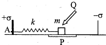
Рис. 3. Пружинный маятник в электрическом поле
