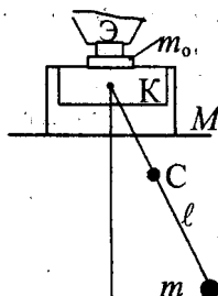
Рис. 5. Маятник с подвижной точкой подвеса
