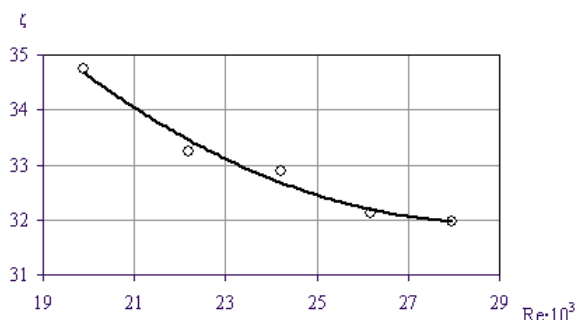
Рис. 4. Зависимость коэффициента гидравлического сопротивления от числа Рейнольдса
