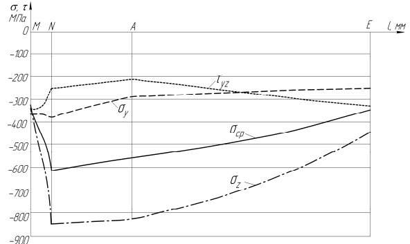
Рис. 5. Компоненты напряжений вдоль правой границы зоны пластичности
