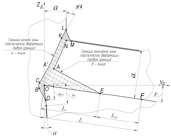
Рис. 1. Схема стружкообразования с развитыми зонами пластической деформации
