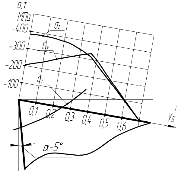
Рис. 6. Распределение контактных напряжений на передней поверхности
