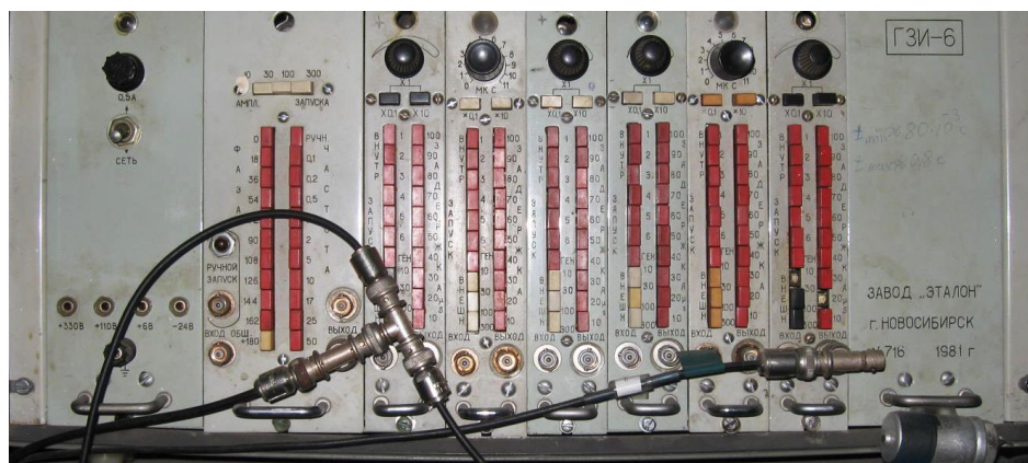
Рисунок 2.8 – 6-канальный генератор импульсов ГИ-1
