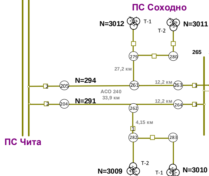
Рисунок А – Схема сетевого участка
