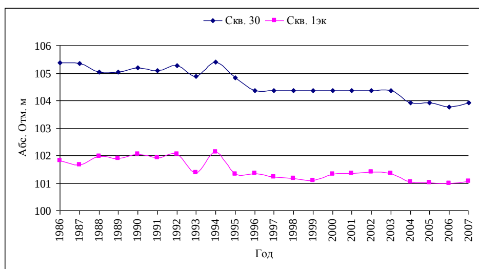
Рисунок 2.1. Графики изменения уровня подземных вод в западной части Лагерного сада (водоносный горизонт палеоген-четвертичных отложений)[11]
