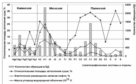
Рис. 1. Связь нефтеобразования с формированием углерод-водородной оболочки, уровнем трансгрессий и распределением числа образцов в БД в фанерозое
