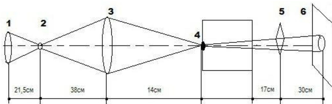
Для более резкого изображения использовался метод лазерного монитора (рис. 3), когда свет от источника проходит через линзу 3, отражается от зеркальной поверхности 1 и проходит обратно через активную среду лазера 4 испустив при этом дополнительные фотоны. Далее световой поток проходит через фильтр 5 и на экране 6 (за счет дополнительных фотонов) формируется более четкое изображение неоднородностей в полупрозрачном теле (рис. 2, б).
