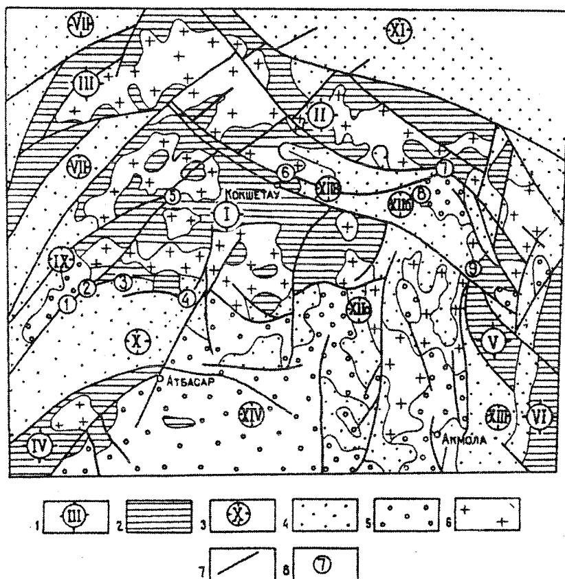
Рис. 1. Тектоническая структура Северо-Казахстанской урановорудной провинции:
