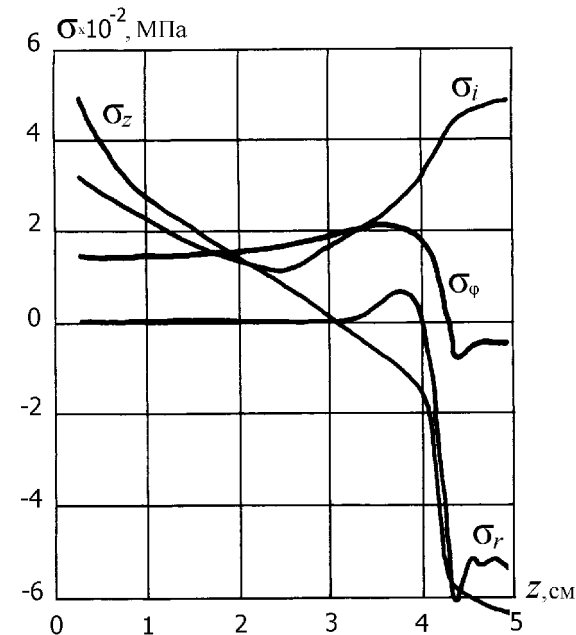
Рис. 2. Распределение напряжений у внутренней поверхности трубы ( r = 7,8 см)
