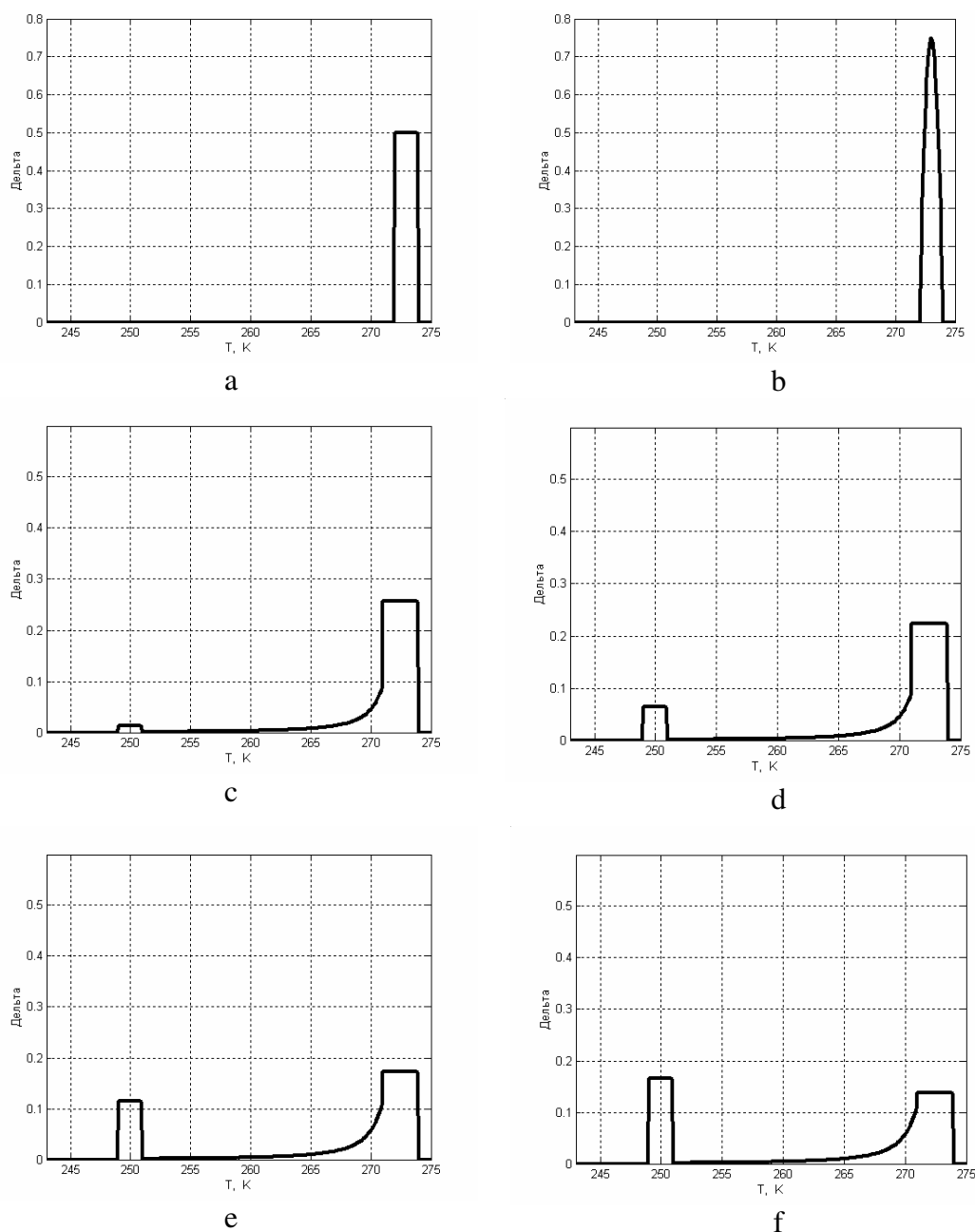
Рис. 2. Плотность распределения источника тепла: а) прямоугольник; б) парабола; в) C_8 = 5 ; д) 15; е) 20; ф) 30 %
