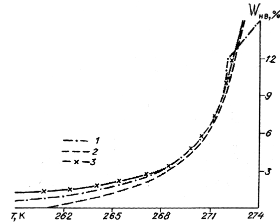
Рис. 1. Сравнение результатов восстановления функции количества незамерзшей воды, полученным численным (1) и кватистиационным (2, 3) методами
