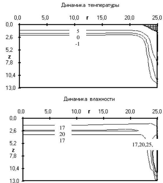
Рис. 3. Распределения температуры и суммарной влажности при C_s=0
