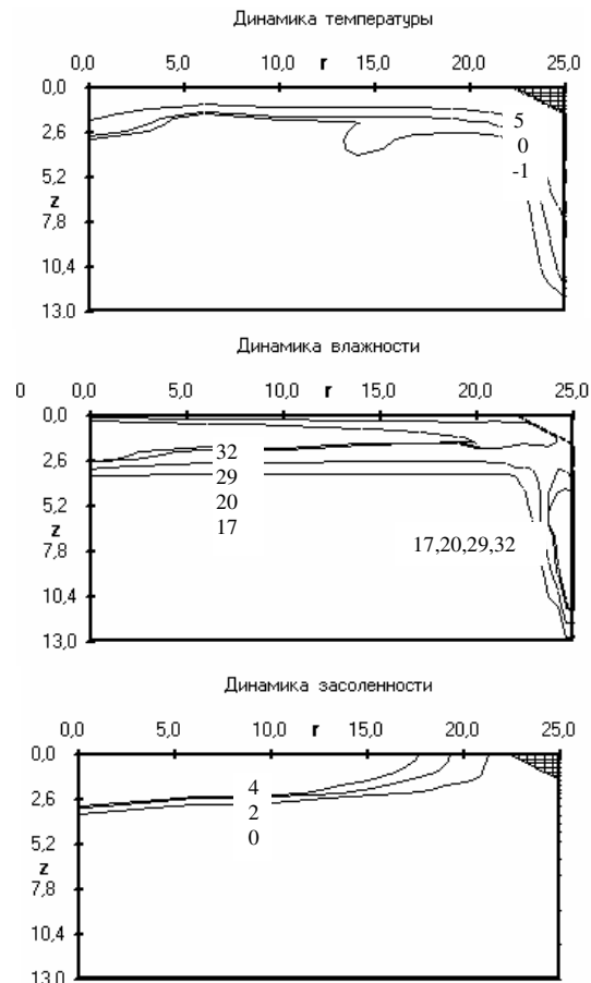
Рис. 4. Распределения температуры, суммарной влажности и засолённости при C_s=100 г/л
