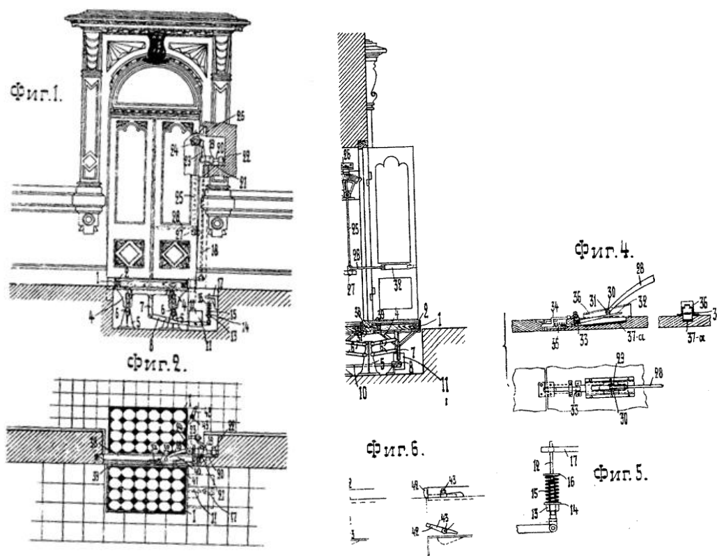
Рисунок 1 – Первое зарегистрированное в СССР устройство автоматического открывания/закрывания дверей
