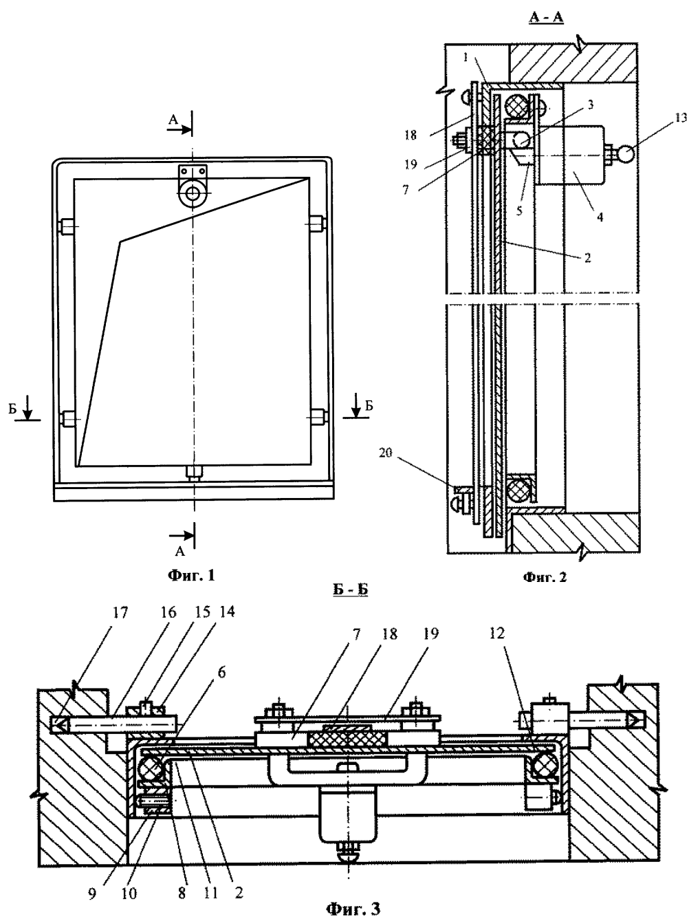
Рисунок 2 – Устройство для дымоудаления
