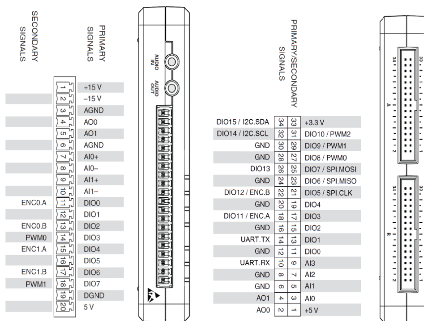
Рисунок 10 – Разъемы и порты NI MyRIO [8]
