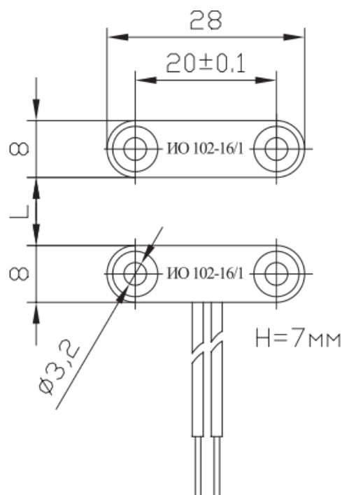
Рисунок 14 – Габаритные размеры магнитоконтактного датчика ИО-102-16/1 [10]
