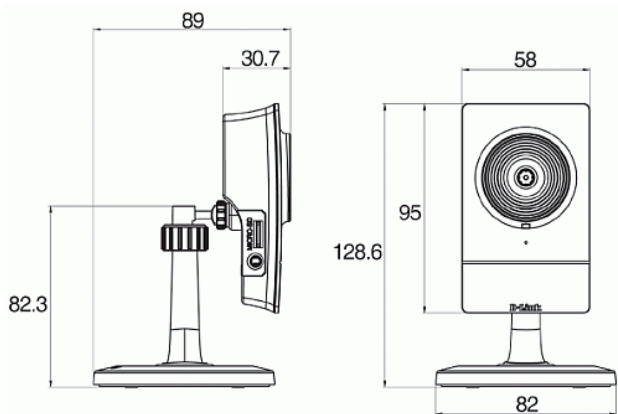
Рисунок 17 – Габаритные размеры камеры D-Link DCS-2103 [12]
