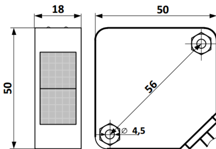
Рисунок 11 – Внешний вид барьерного датчика ВИКО-Б-109-ПЗ [9]
